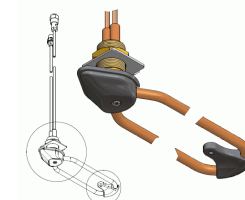
KEEL COOLER FOR AC UNIT
