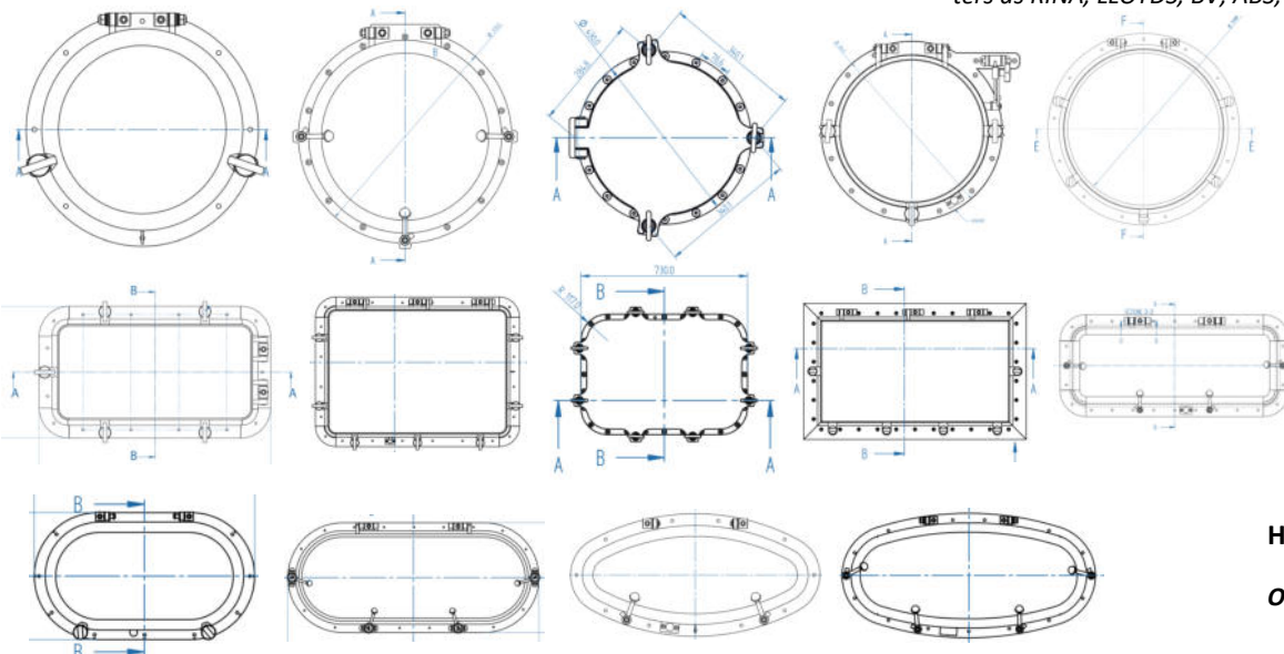
Kiểu tròn
