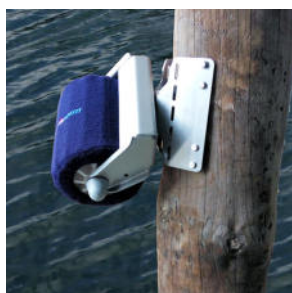
Tấm chắn dạng cuộn cho cột với trục xoay Roller bumper for pillar, pivoting
