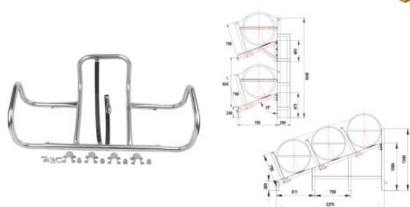
Khung đỡ bè cứu sinh
